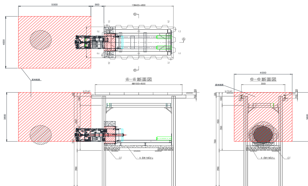
図5. 開削による造成径確認予定図
