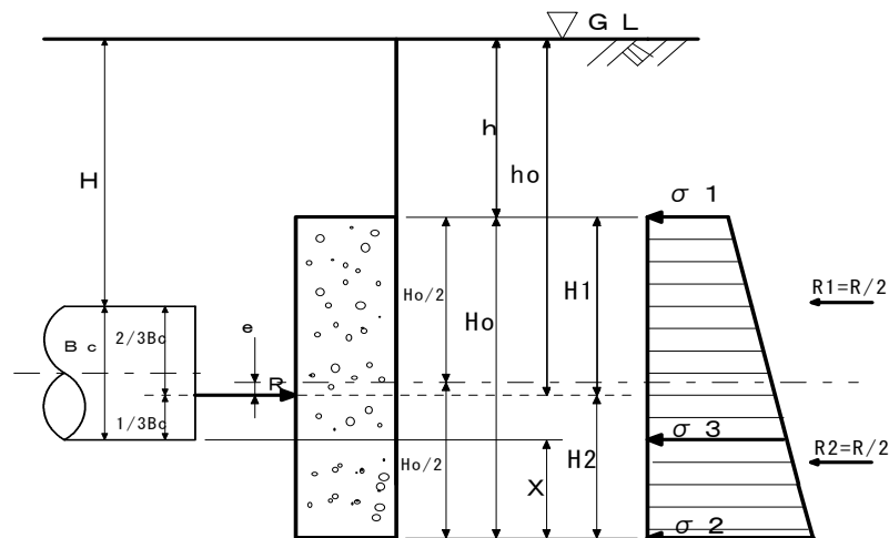
支圧壁の計算図
