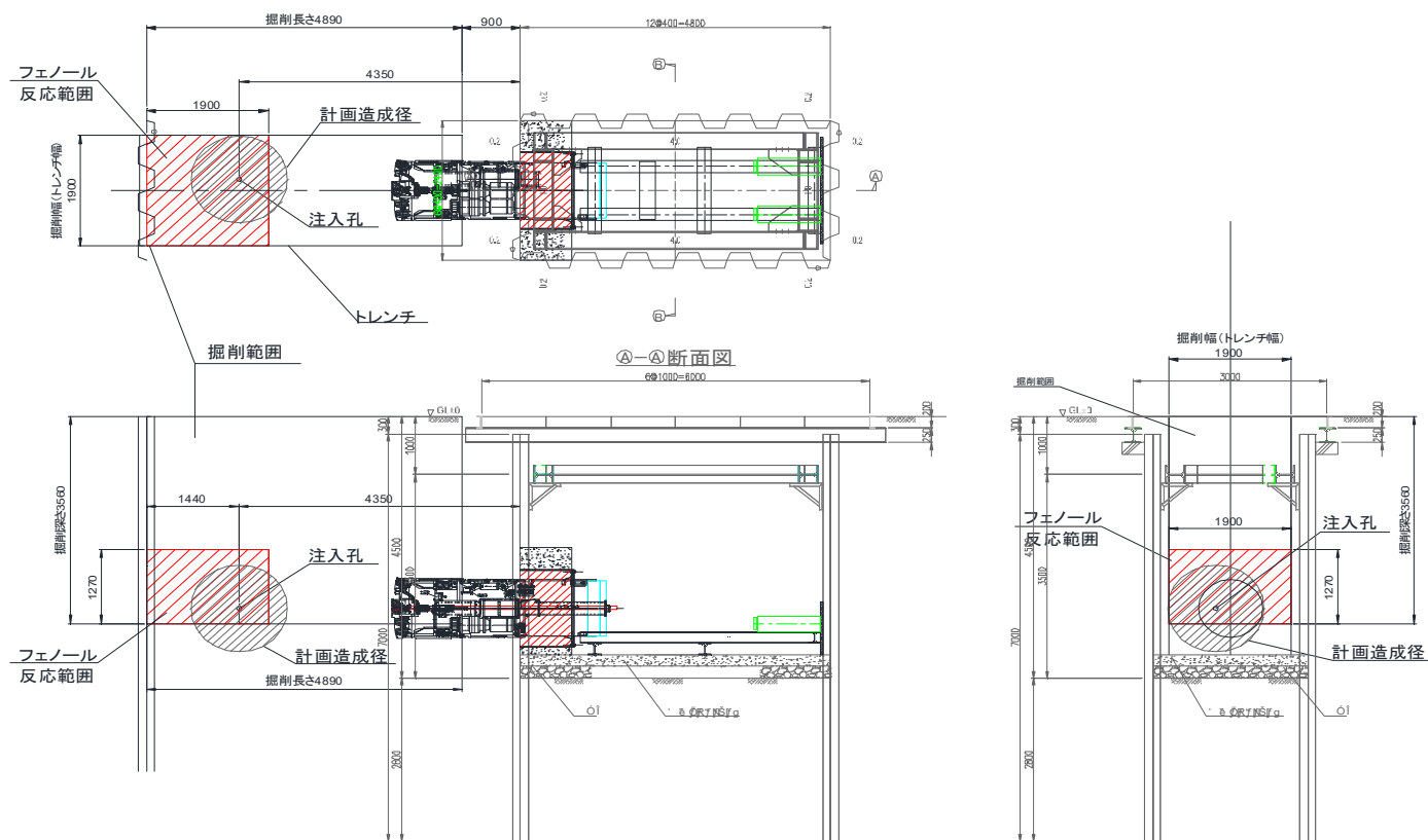
図6. 開削による造成径確認結果図
