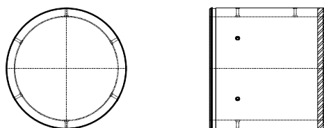
φ 2200mm注入管（注入孔6箇所）
