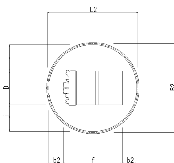
到達立坑図(ライナー参考)
