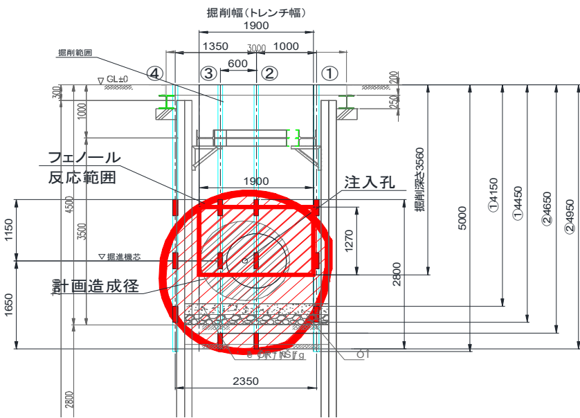
図7. ボーリング調査及び開削による造成径確認合成図（幅、高）
