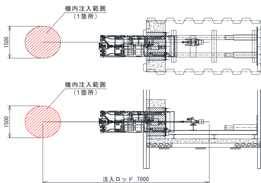
図1. 機内注入実験施工図
