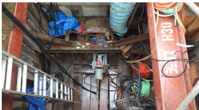
写2. 機内注入工法施工状況②（立坑内状況）
