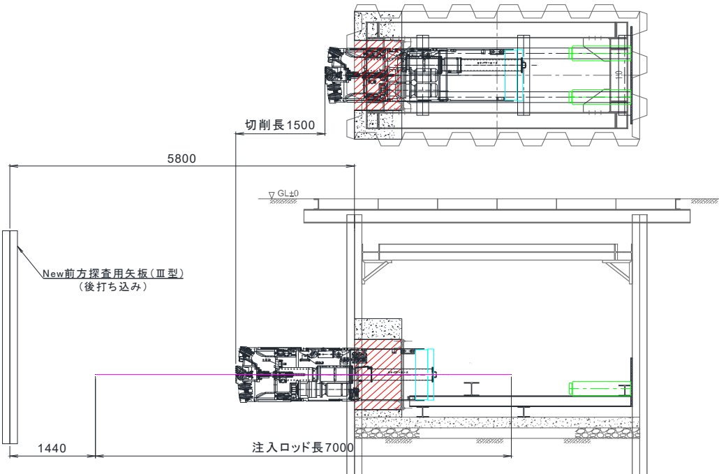
図2. 注入位置図
