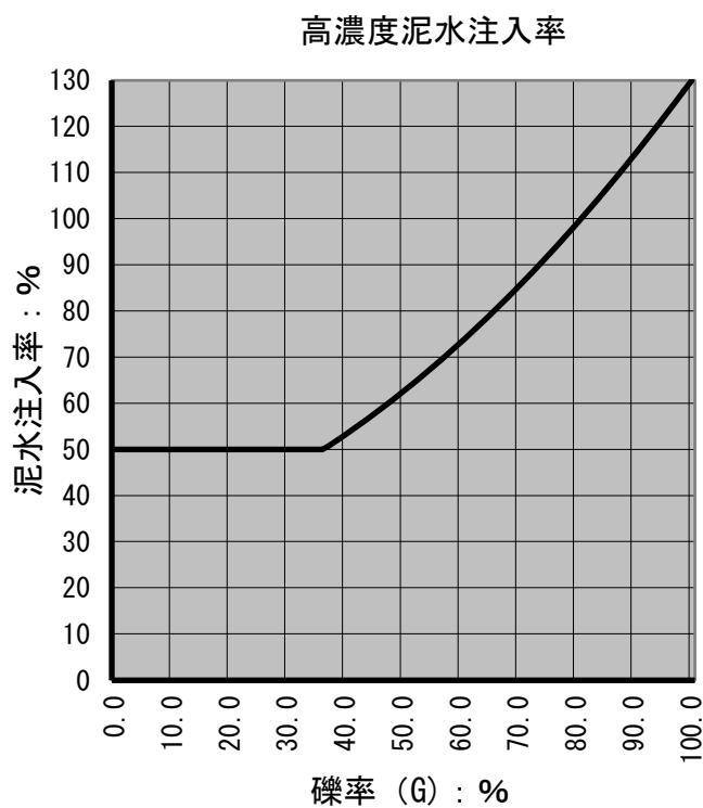
高濃度泥水注入率(土質C、Cq:参考)
