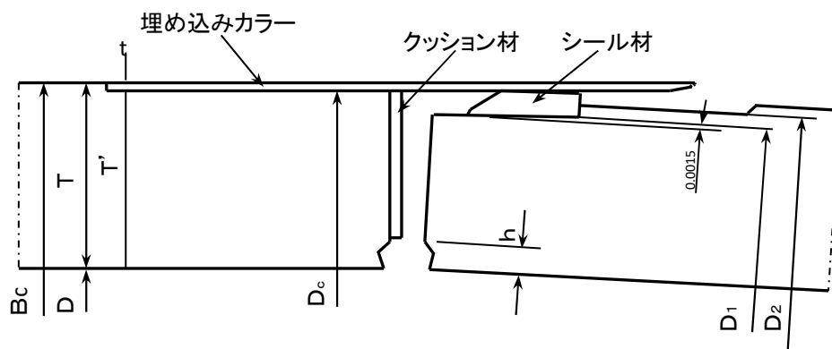
継手部詳細
