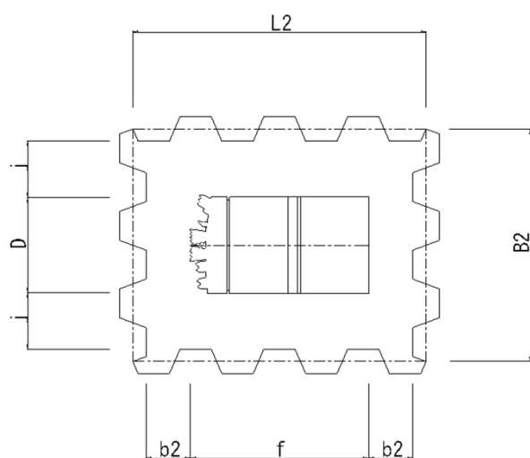
到達立坑図(Ⅲ鋼矢板参考)
