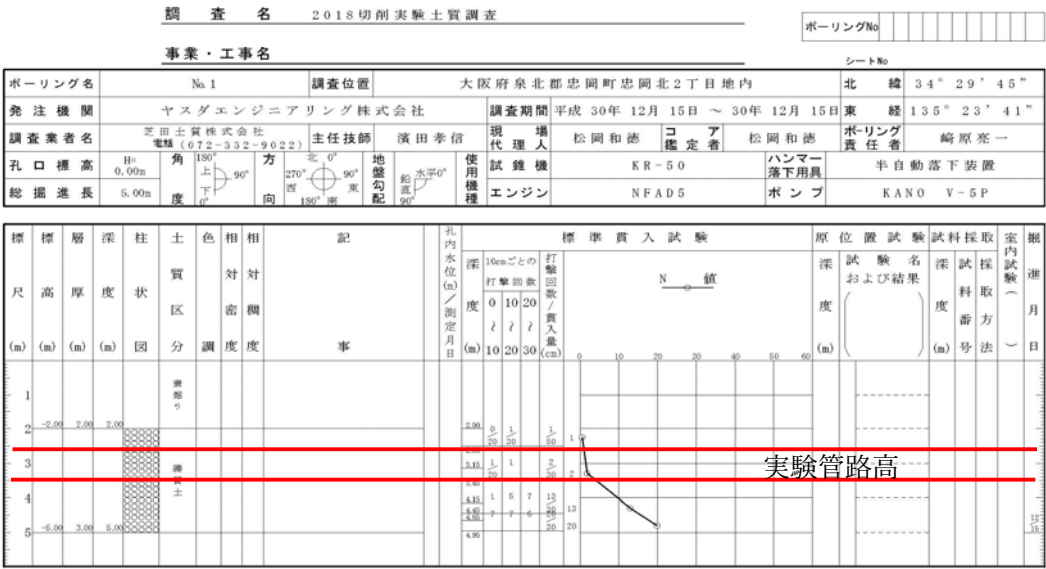
ボーリング柱状図
