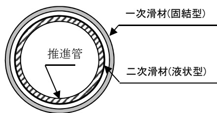
縁切り層の形成方式
