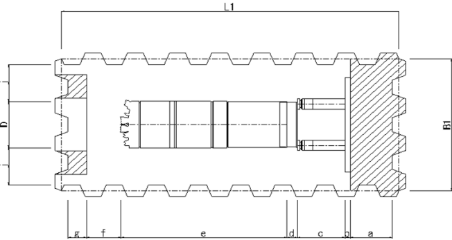
発進立坑図(鋼矢板参考)
