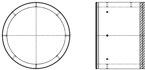
φ 3000mm注入管（注入孔8箇所）
