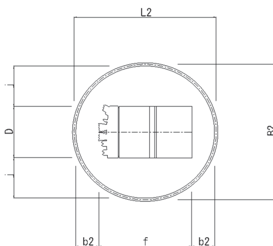
到達立坑図(ライナー参考)
