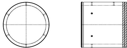
φ 2200mm注入管（注入孔6箇所）
