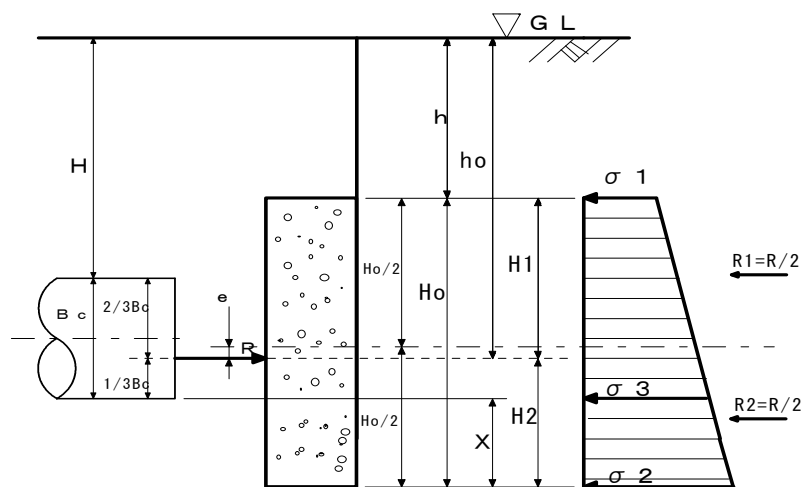
支圧壁の計算図
