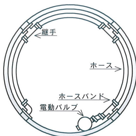
注入管の配管方法（4孔管の場合）
